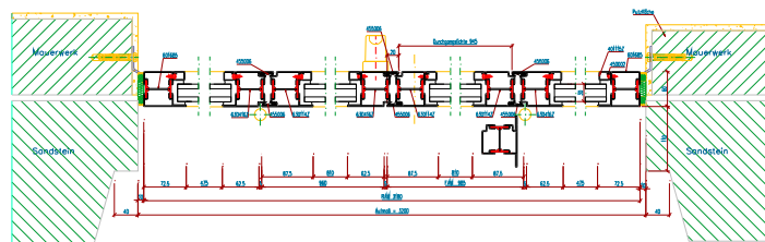
H-Schnitt
